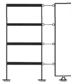
(c) 摇摆墙结构体系(墙底铰接)
