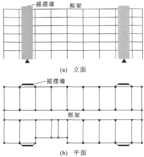
图 5 工况 1 的摇摆墙布置
