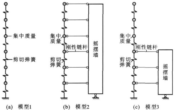
图 6 计算模型
